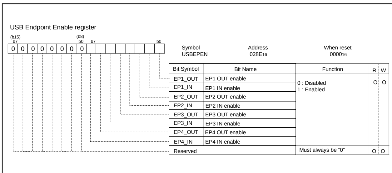
Figure 2.8.11. USB endpoint enable register
