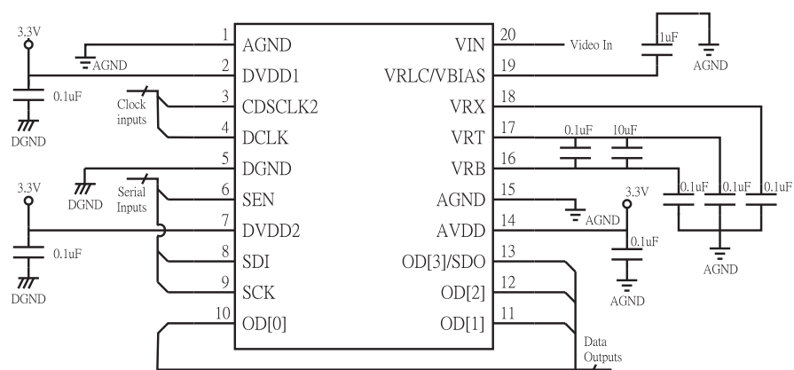
HT82V42 SSOP-20
