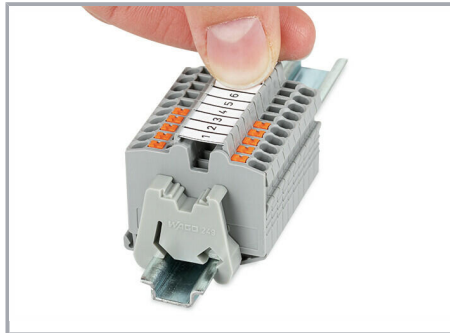
Einrasten eines Beschriftungsstreifens (2009-110) in die Beschriftungsaufnahme
