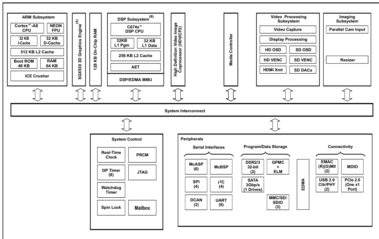
图 1-1. TMS320DM814x DaVinci™ 视频处理器功能方框图
