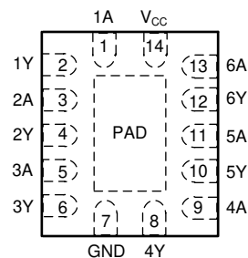
图 4-2. BQA 封装，14 引脚 WQFN ( 顶视图 )
