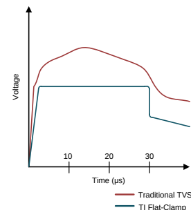
对 8/20μs 浪涌事件的电压钳位响应
