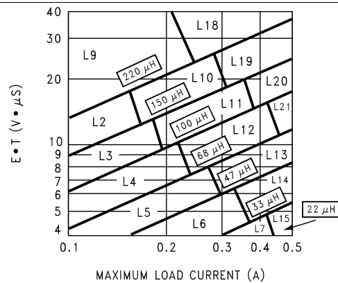
Figure 20. LM2671-ADJ
