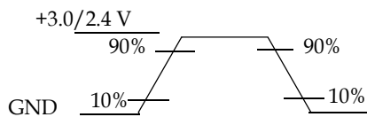
Figure A: Input Waveform
