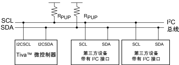
图 16-2. I 2 C 总线配置
