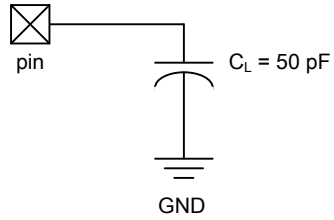
图 22-1. Load Conditions
