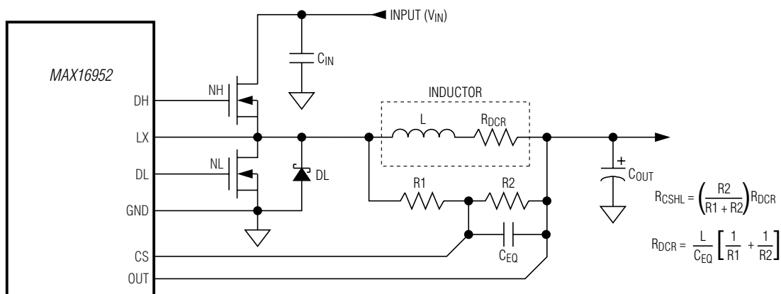
b) LOSSLESS INDUCTOR SENSING
