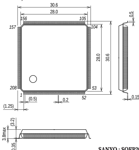
外形図 3210 (unit : mm)
