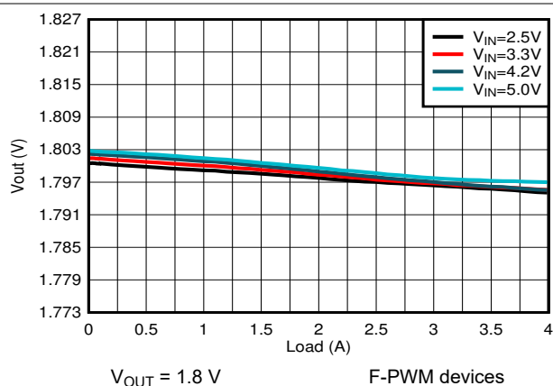
图 9-14. Load Regulation
