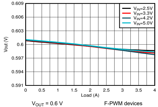
图 9-6. Load Regulation
