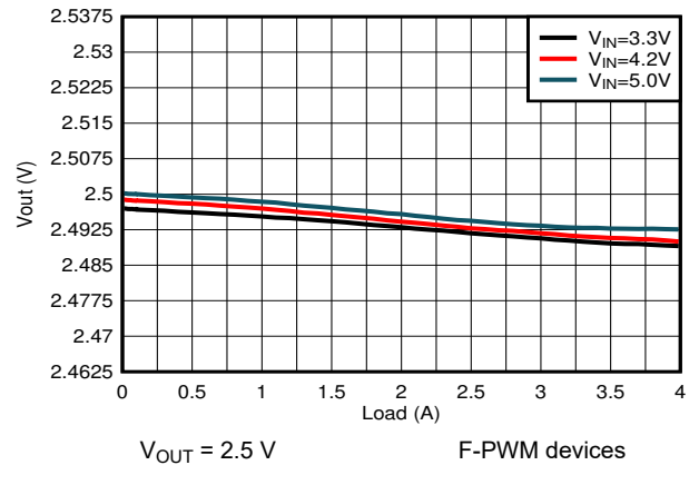
图 9-18. Load Regulation
