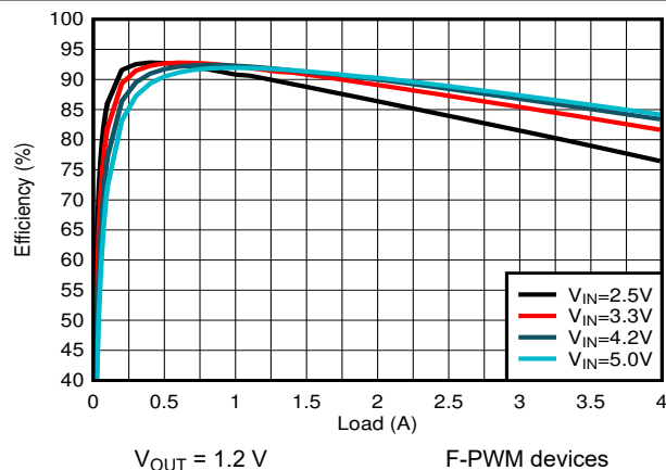
图 9-9. PWM Efficiency
