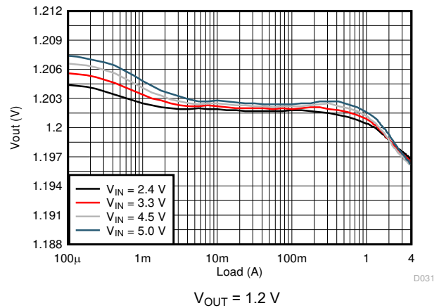
图 9-8. Load Regulation
