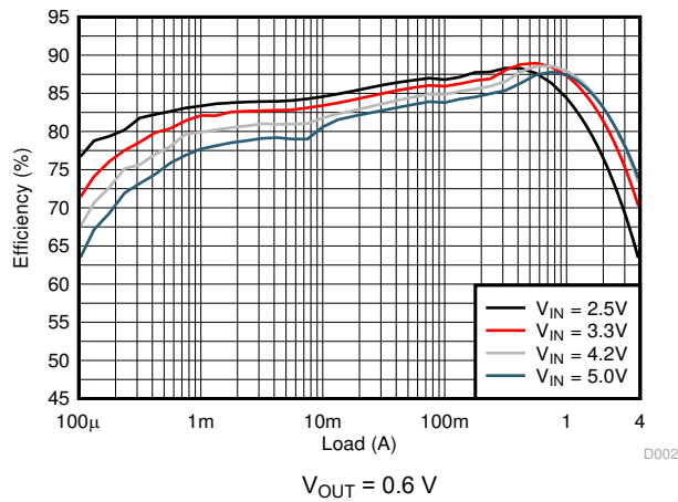
图 9-3. Efficiency
