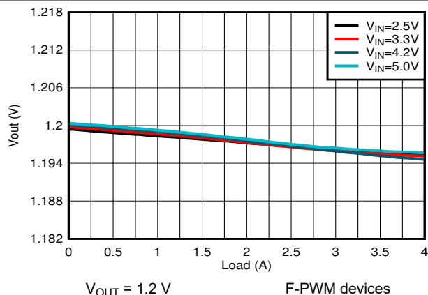
图 9-10. Load Regulation
