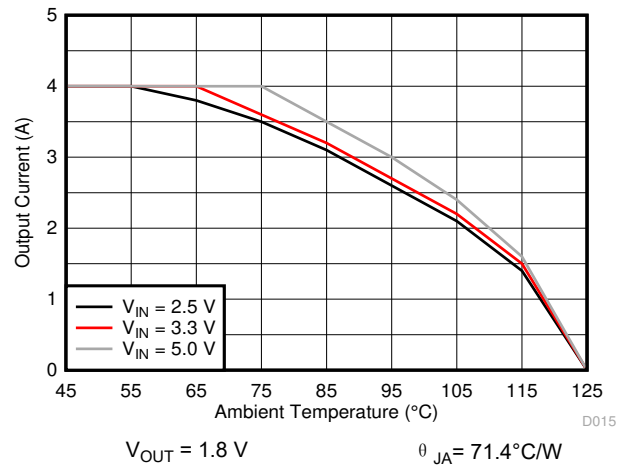
图 9-30. Thermal Derating
