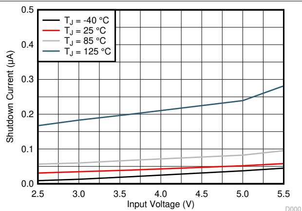
图 7-3. Shutdown Current
