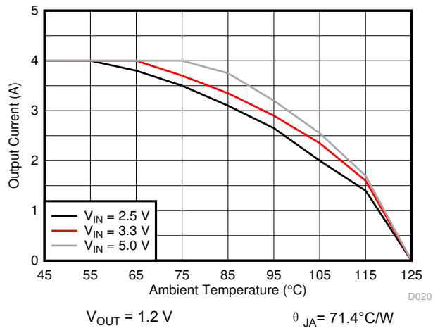
图 9-29. Thermal Derating
