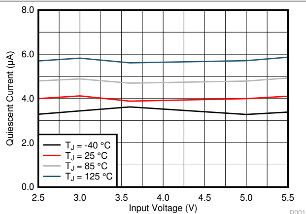
图 7-4. Quiescent Current
