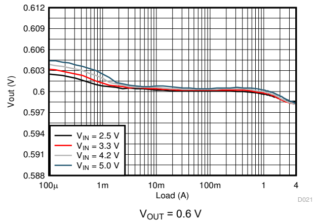
图 9-4. Load Regulation
