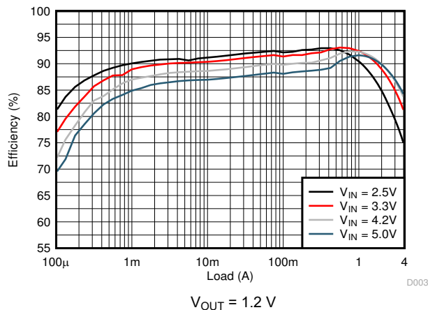
图 9-7. Efficiency
