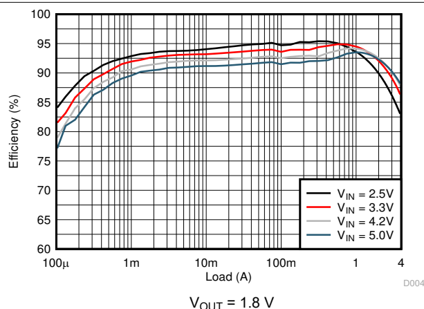
图 9-11. Efficiency
