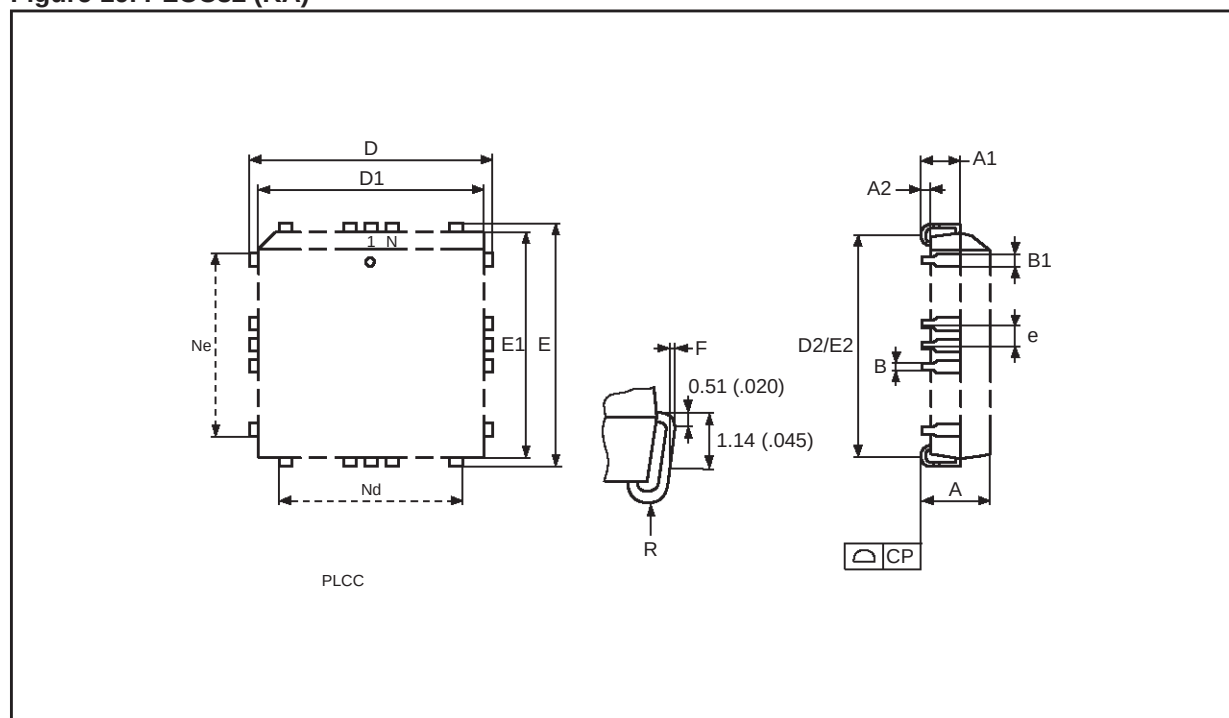
Figure 19. PLCC32 (KA)
