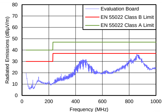
辐射电磁干扰 (EMI) (CISPR22) V_{IN} = 5.0V 、 V_{OUT} = 1.8V 、 I_{OUT} = 650mA
