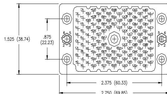
120 PIN RECEPTACLE
