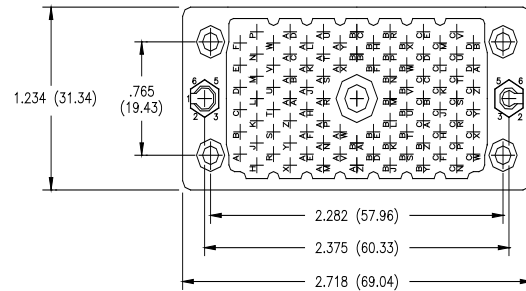
120 PIN RECEPTACLE
