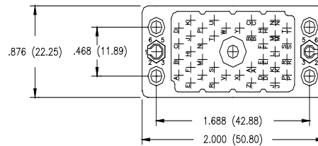
38 PIN RECEPTACLE
