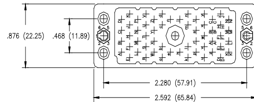
56 PIN RECEPTACLE
