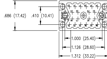
20 PIN RECEPTACLE
