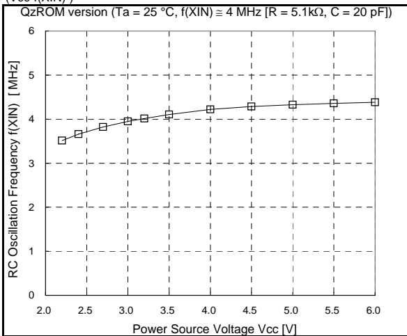
Fig. 44. Vcc-f(XIN)
