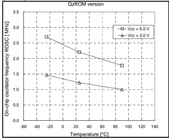
Fig. 41. Ta-Rosc
