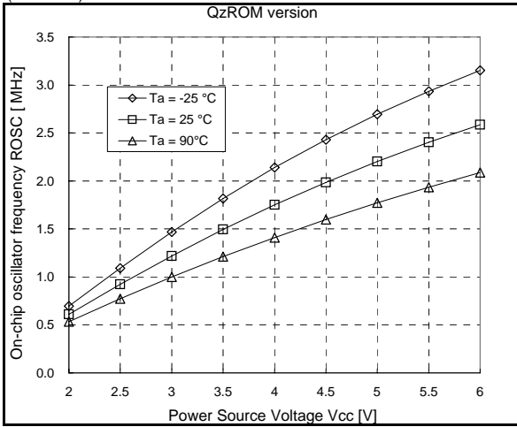
Fig. 40. Vcc-Rosc
