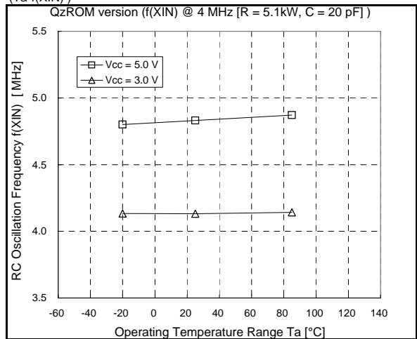
Fig. 45. Ta-f(XIN)
