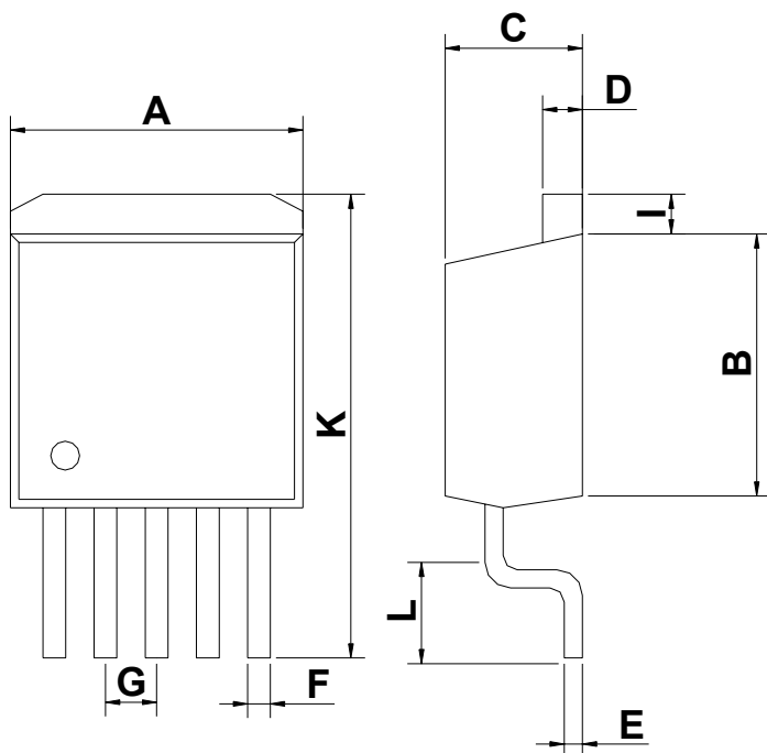
TO-263 (N263)
