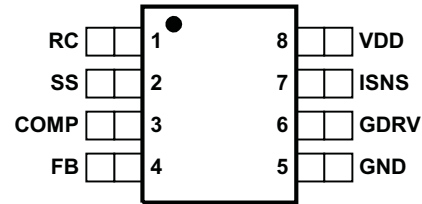
8 PINS SOIC (D) PACKAGE (TOP VIEW)
