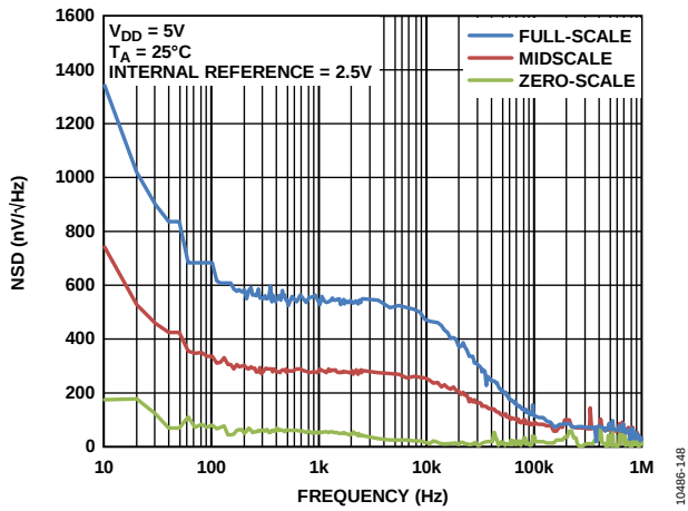
图41. 噪声频谱密度
