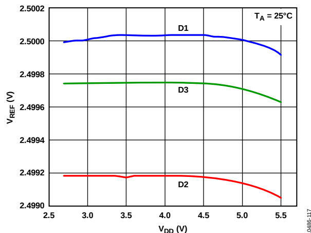
图11 内部基准电压与电源电压的关系
