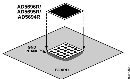
图57. 焊盘与电路板的连接
