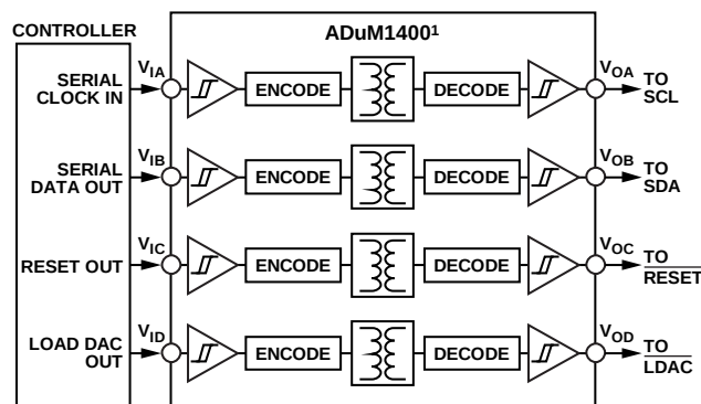
图58. 隔离接口
