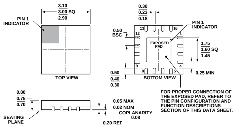
图59. 16引脚引脚架构芯片级封装[LFCSP_WQ]
