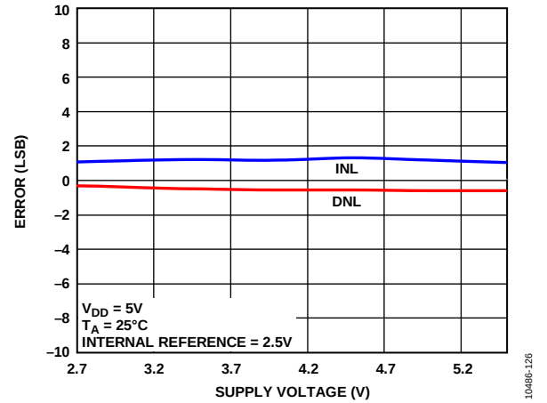
图20. INL误差和DNL误差与电源电压的关系
