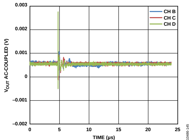
图38. 模拟串扰(通道A)
