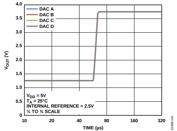
图34. 建立时间(5.25 V)
