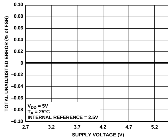
图26. TUE与电源的关系(增益=1)
