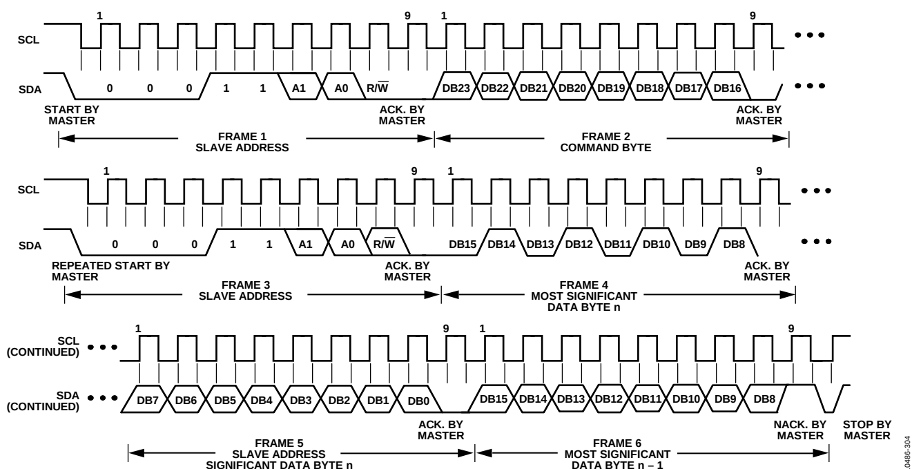
图51. I²C读操作
