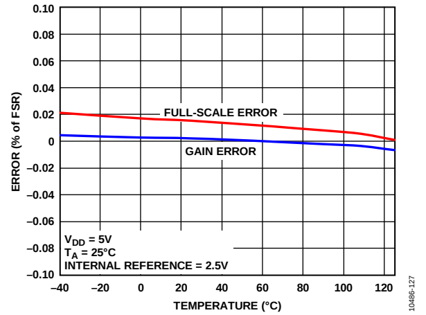
图21. 增益误差和满量程误差与温度的关系
