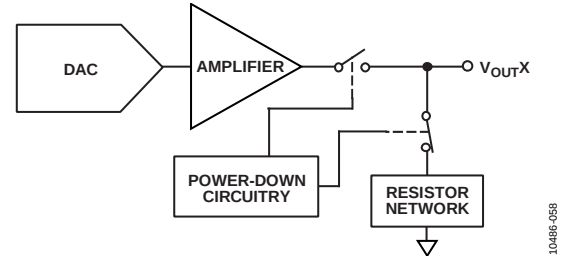
图52. 掉电模式下的输出级
