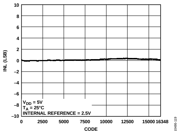
图13. AD5695R INL
