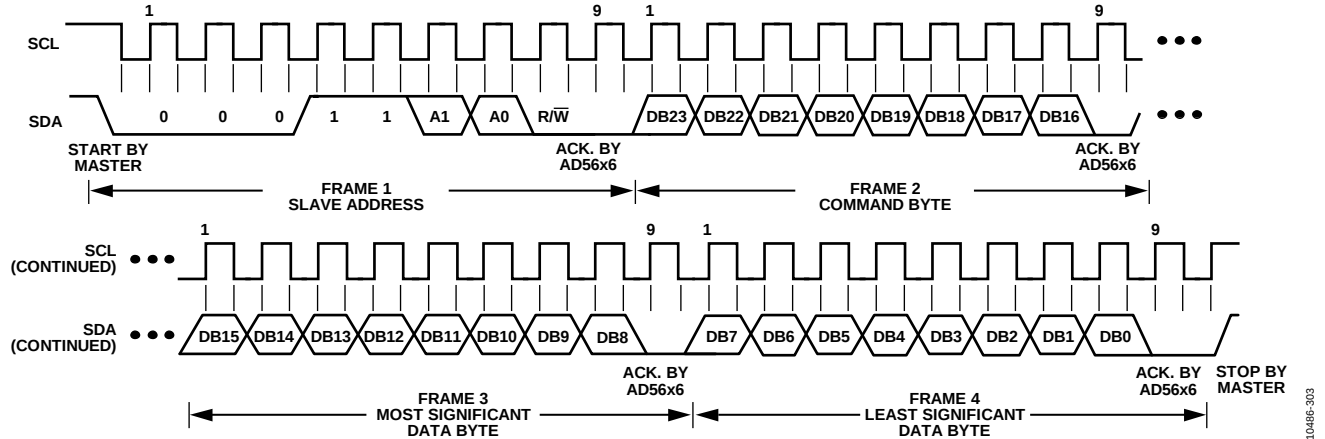
图50. I²C写操作
