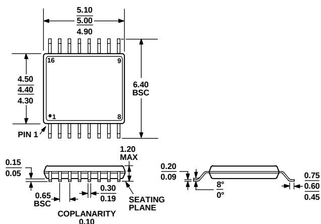
图60. 16引脚超薄紧缩小型封装[TSSOP]
