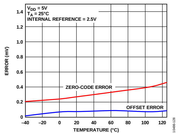
图22. 零代码误差和失调误差与温度的关系
