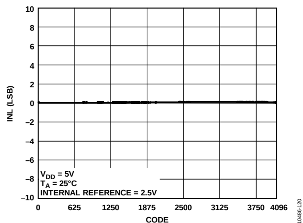
图14. AD5694R INL
