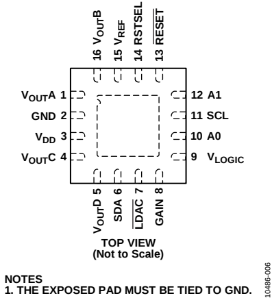
图3. 16引脚LFCSP的引脚配置
