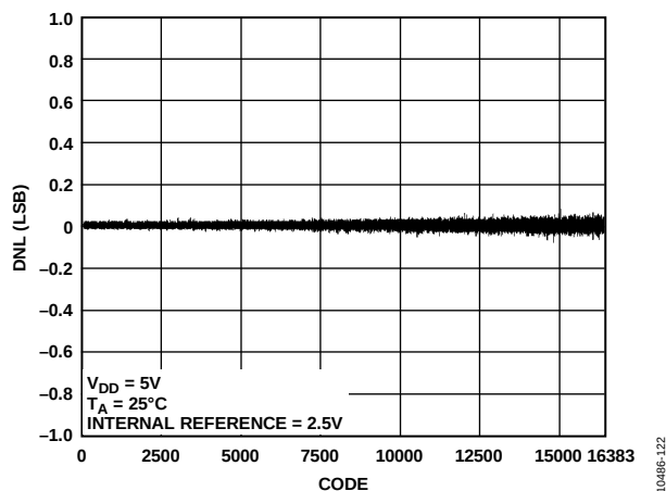
图16. AD5695R DNL
