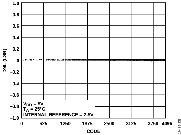
图17. AD5694R DNL
