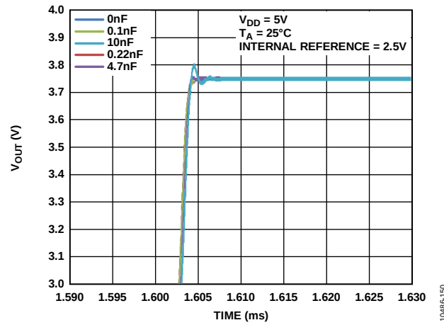
图43. 建立时间与容性负载的关系
