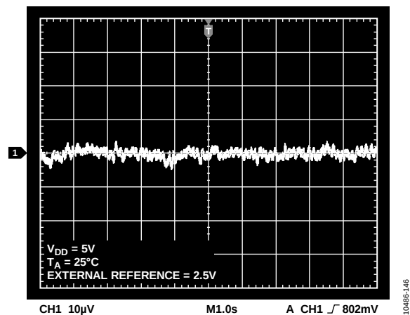
图39. 0.1 Hz至10 Hz输出噪声图，外部基准电压源
