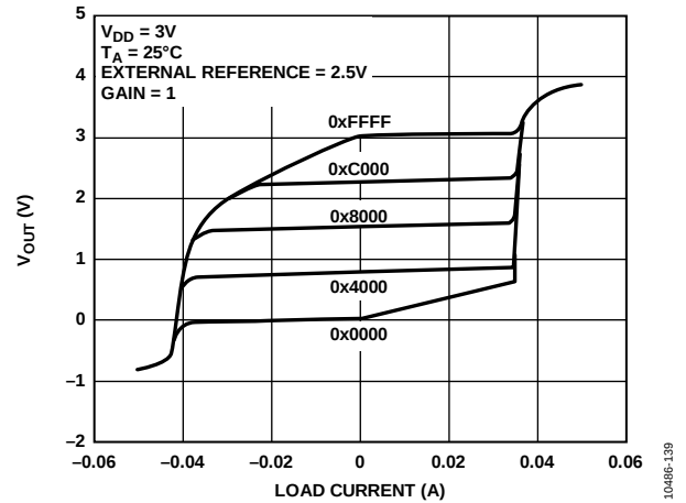
图32. 3 V时的源电流和吸电流能力
