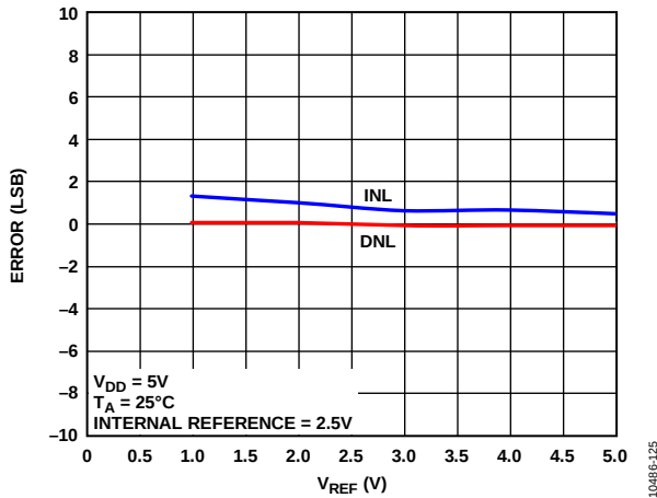
图19. INL误差和DNL误差与 V_{REF} 的关系
