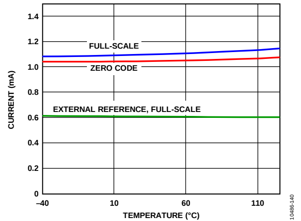
图33. 电源电流与温度的关系
