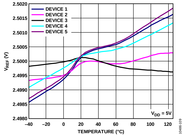
图6. 内部基准电压与温度的关系(A级)
