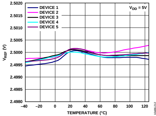
图5. 内部基准电压与温度的关系(B级)
