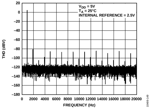
图42. 1 kHz时的总谐波失真
