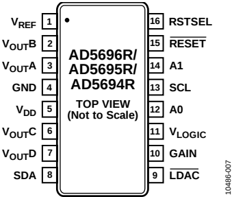
图4. 16引脚TSSOP引脚配置
