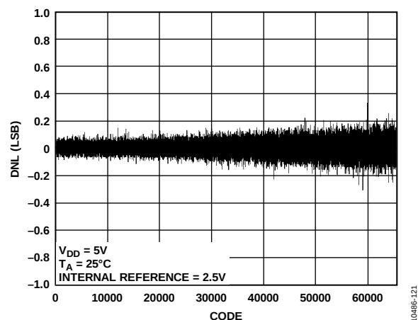
图15. AD5696R DNL
