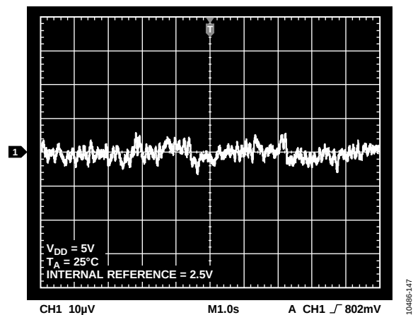
图40. 0.1 Hz至10 Hz输出噪声图，2.5 V内部基准电压源
