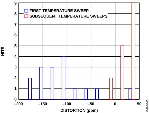
图55. 热滞
