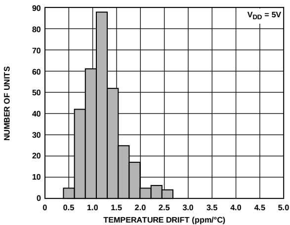
图7. 基准电压输出温度漂移直方图
