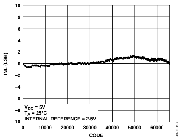
图12. AD5696R INL
