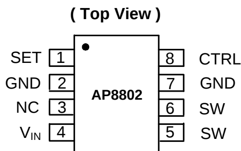
(1) SOP-8L
