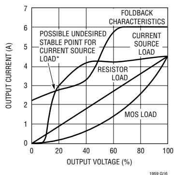
电流限值折返
