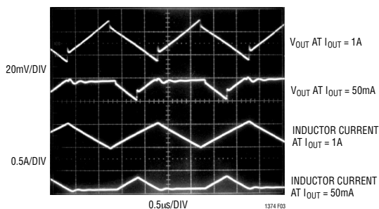
图 3：LT1959 纹波电压的波形
