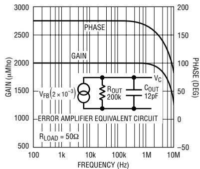
误差放大器跨导
