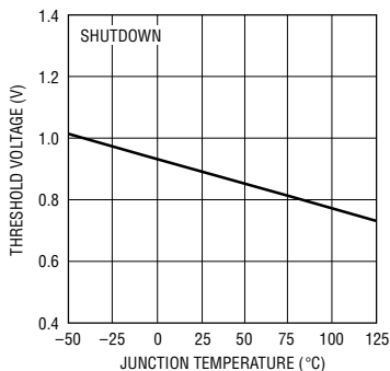
V_C 引脚关断门限
