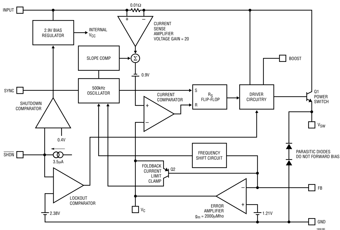
图 1：方框图
