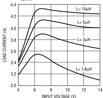
V_{OUT} = 3.3V 时的最大负载电流
