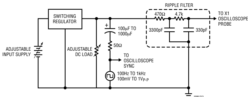
图 13：环路稳定性测试电路
