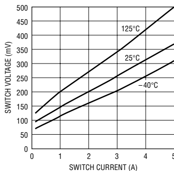
开关管的压降
