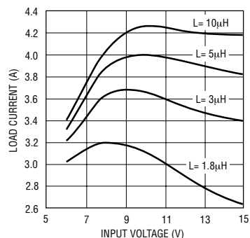
V_{OUT} = 5V 时的最大负载电流
