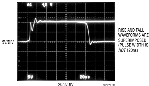
图7: 开关节点的共振
