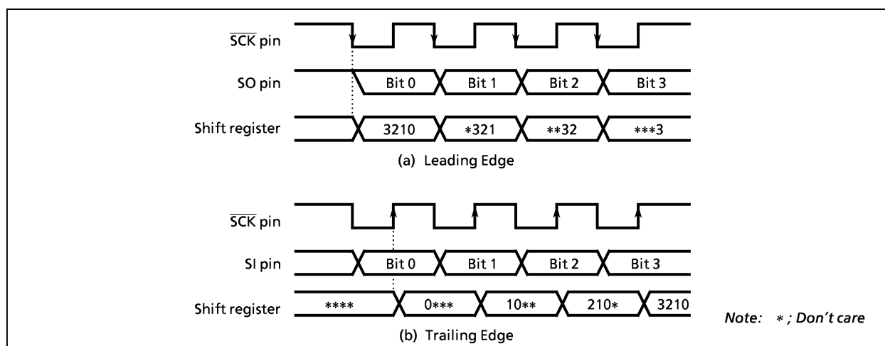
Figure 2-36. Shift Edge
