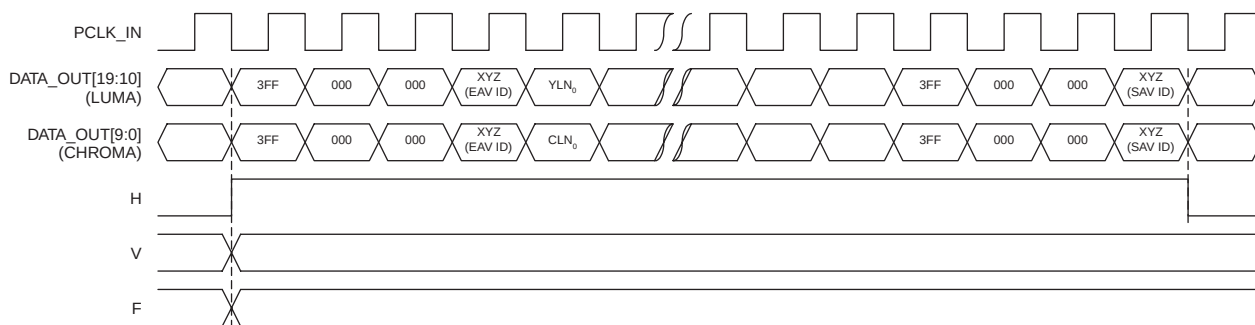
Fig. 2 HVF Timing
