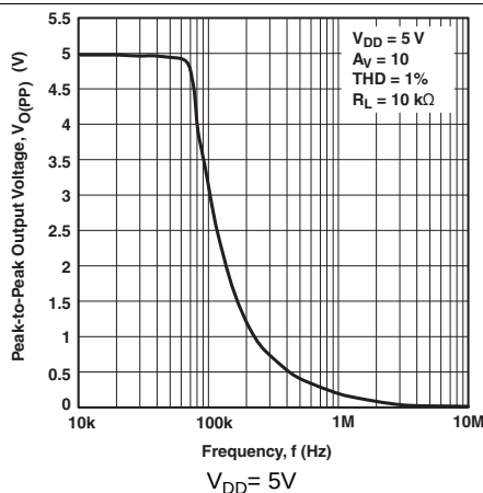
图 10. 峰间输出电压与频率间的关系
