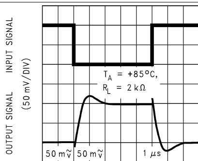
TIME (1 \mu s/DIV) 图 45. 反相小信号脉冲响应
