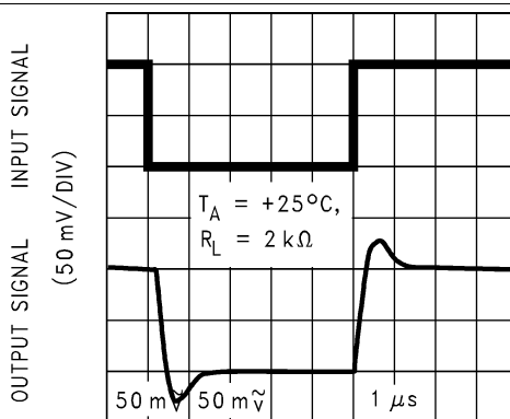
TIME (1 \mu s/DIV) 图 50. 同相小信号脉冲响应
