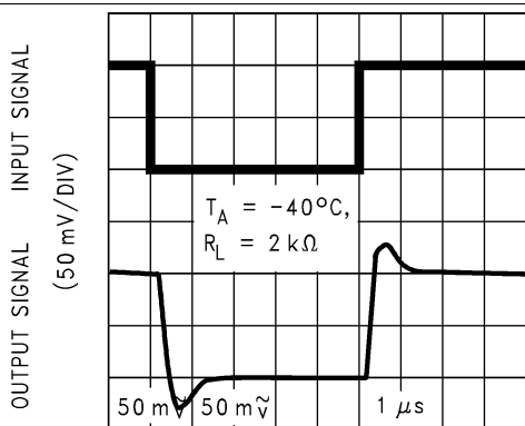
TIME (1 \mu s/DIV) 图 49. 同相小信号脉冲响应
