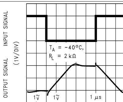
TIME (1 \mu s/DIV) 图 46. 反相大信号脉冲响应
