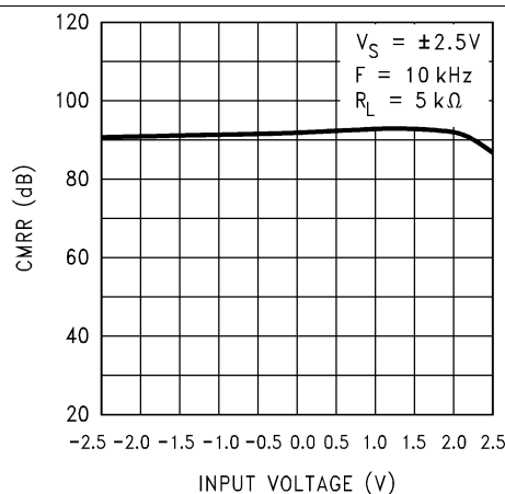
图 20. CMRR 与输入电压间的关系
