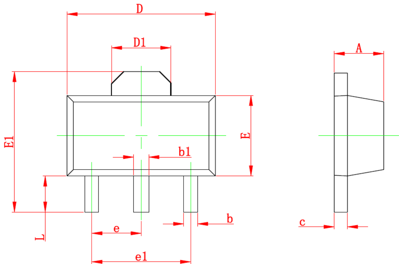
SOT89-3 封装外形尺寸:
