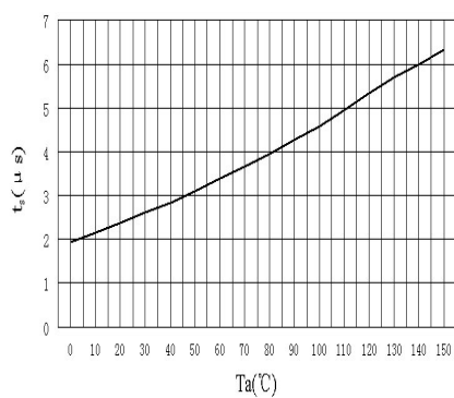
t_S - T_A
