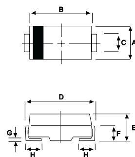
DO-214AC(SMA)
