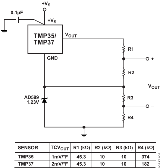
图25. TMP35/TMP37华氏温度计
