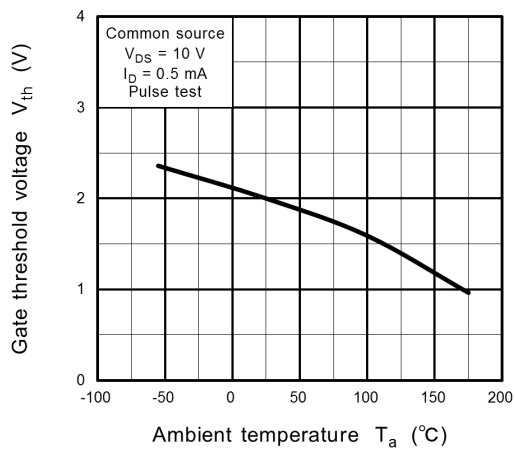
Fig. 8.9 V_{th} - T_a
