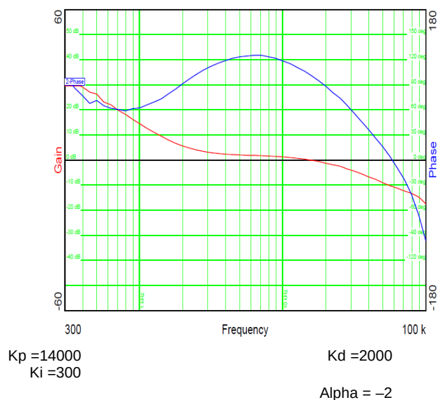
图 7-12. Bode Plot
