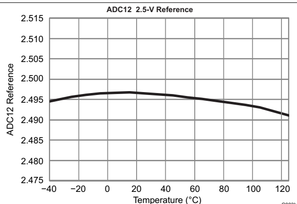
图 5-7. ADC12 2.5-V Reference vs Temperature
