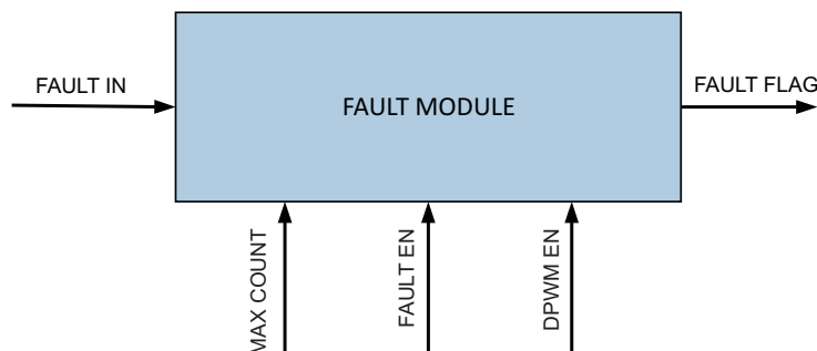
图 6-18. Fault Module
