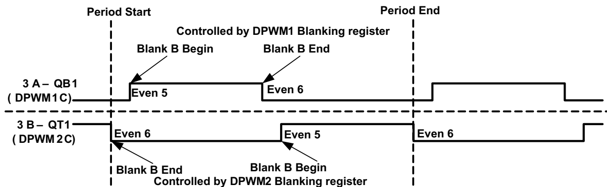
图 7-5. Blank B Timing Information
