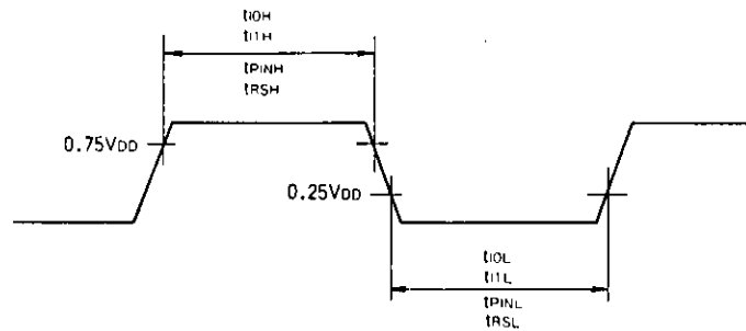
Fig. 7 \text{INT0} , \text{INT1} , \text{INT2} , \text{PIN1} , \text{RES} Input Timing
