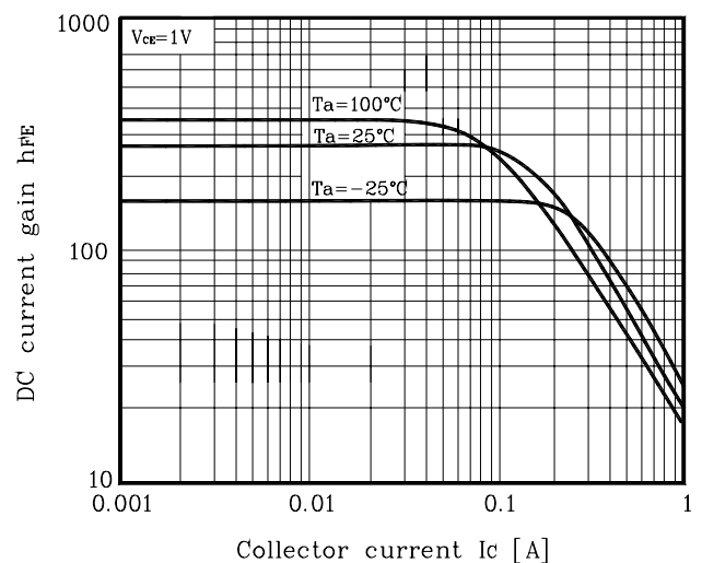
Fig. 6 h_{FE} - I_C
