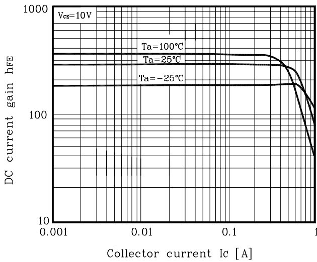
Fig. 9 h_{FE}-I_C
