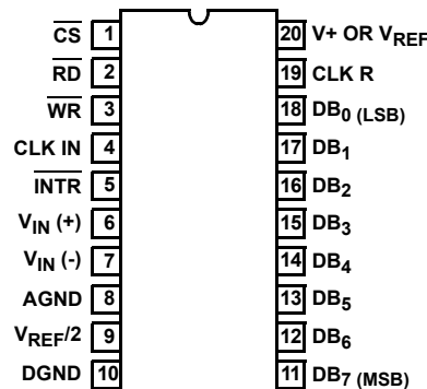
ADC0803, ADC0804 (PDIP)
