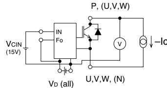
Fig. 2 V_{EC} Test
