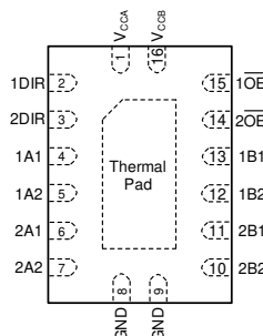
图 5-2. BQB 封装 16 引脚 WQFN 透明顶视图
