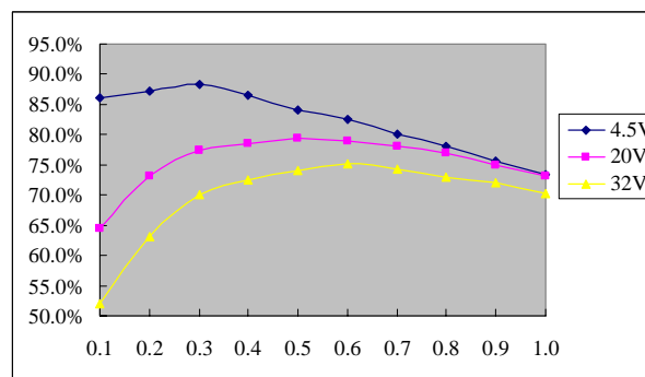
Vo = 1.2V
