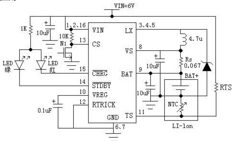
图 1 HM5065 为 4.2V 锂离子电池 1.5A 充电 (150mA 预充) 应用示意图
