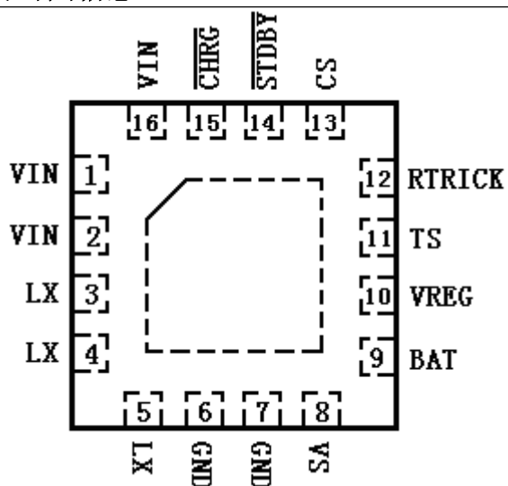
16 引脚 4mm*4mmQFN16 封装顶视图
