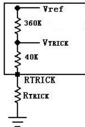
图 7 TRICK 端口内部电路图
