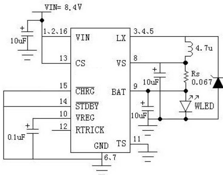
图 12 HM5065 为两接锂电驱动 5W WLED 应用示意图 (RTRICK 引脚悬空)
