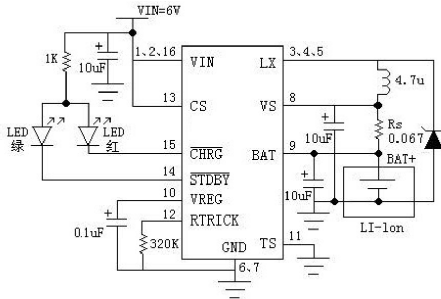
图 10 HM5065 为 4.2V 锂离子电池无电池温度保护涓流 0.75A 恒流 1.5A 充电应用示意图 (CS 引脚接高)
