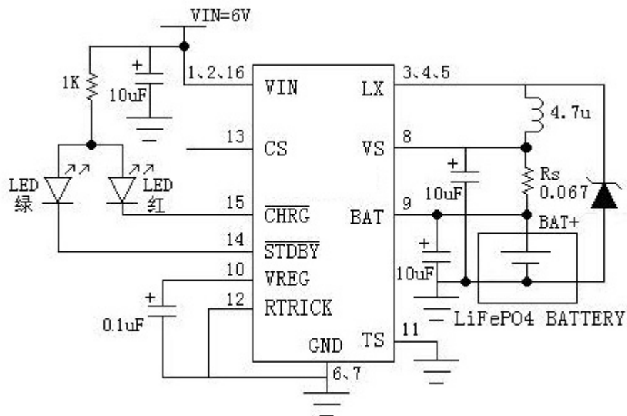
图 11 HM5065 为磷酸铁锂电池无电池温度保护 1.5A 充电应用示意图 (CS 引脚悬空)
