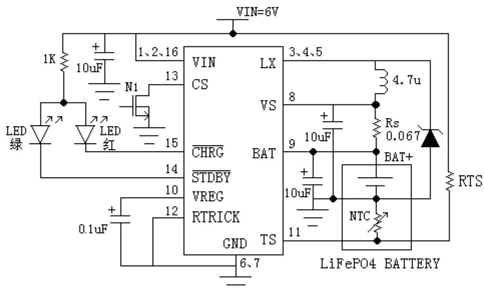
图 2 HM5065 为 3.6V 磷酸铁锂电池 1.5A 充电 (150mA 预充) 应用示意图
