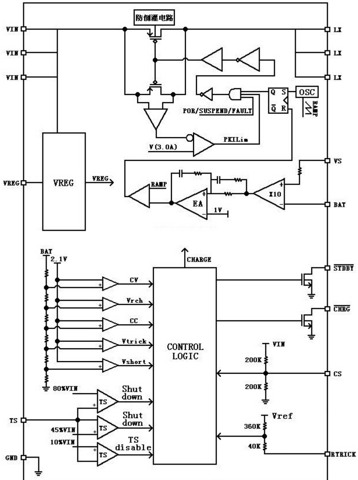
图 3 HM5065 功能框图
