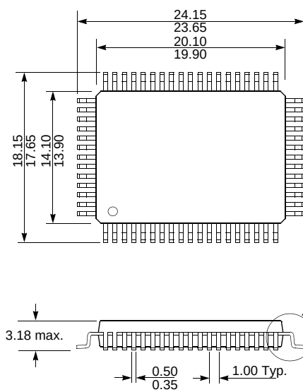
64MQFP
