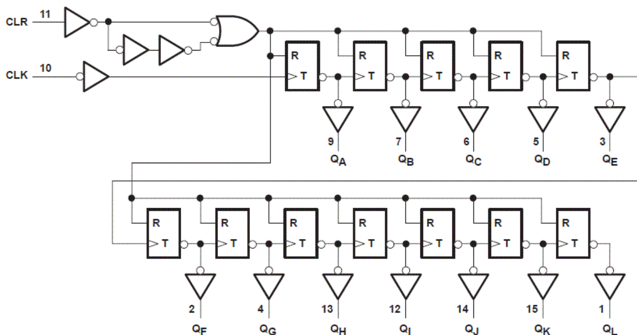
功能框图
