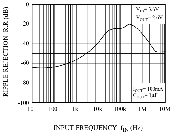
f_{IN} - R.R (7)
