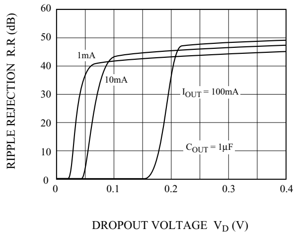
V_D - R.R (1)
