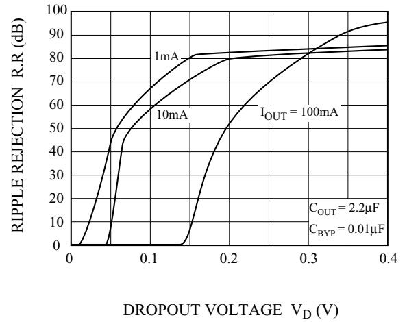
V_D - R.R (2)
