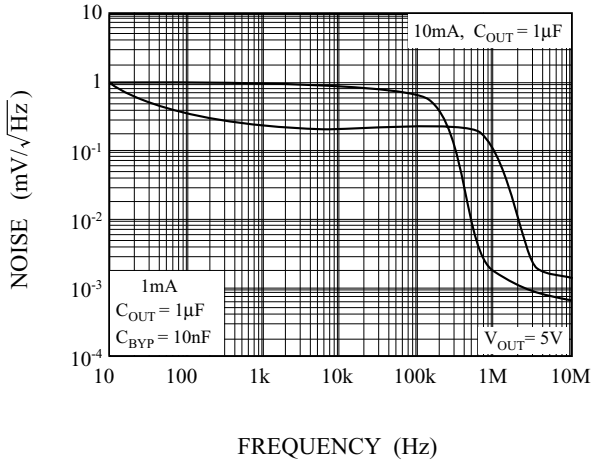
f - NOISE (1)
