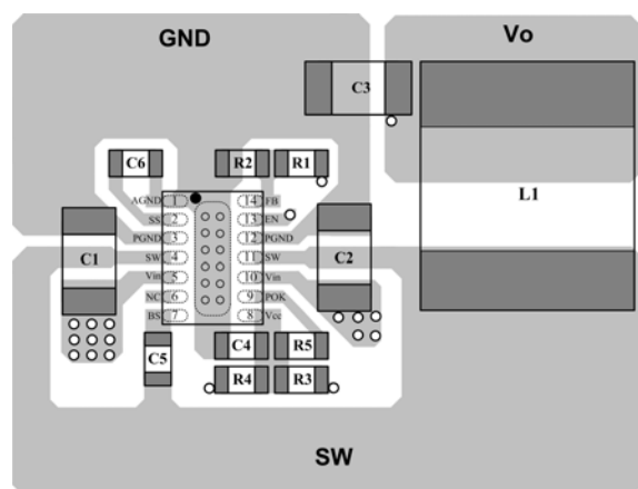
Top layer
