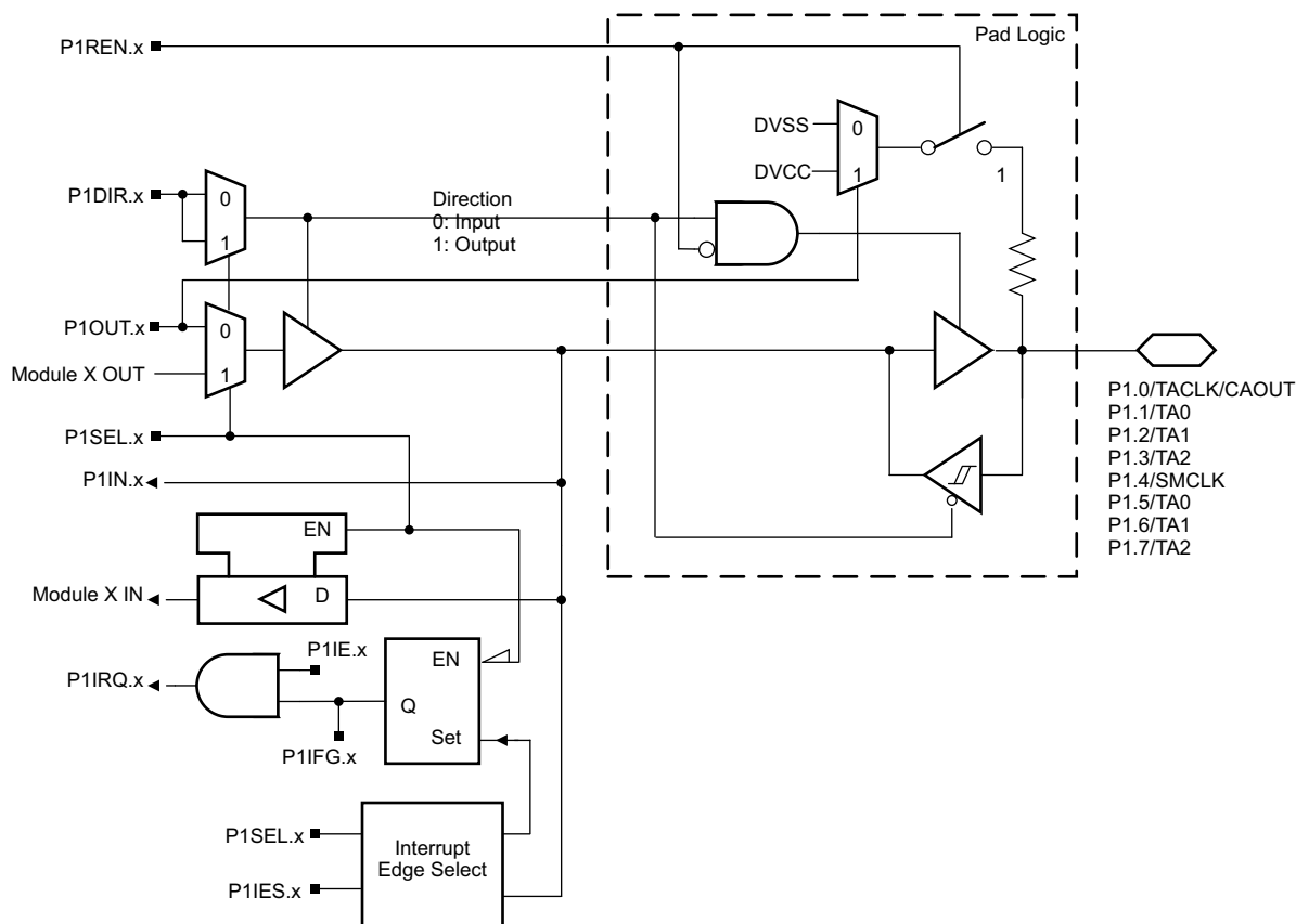
图 9-6. Port P1 (P1.0 to P1.7) Diagram
