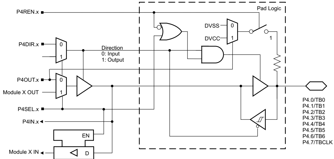
图 9-10. Port P4 (P4.0 to P4.7) Diagram
