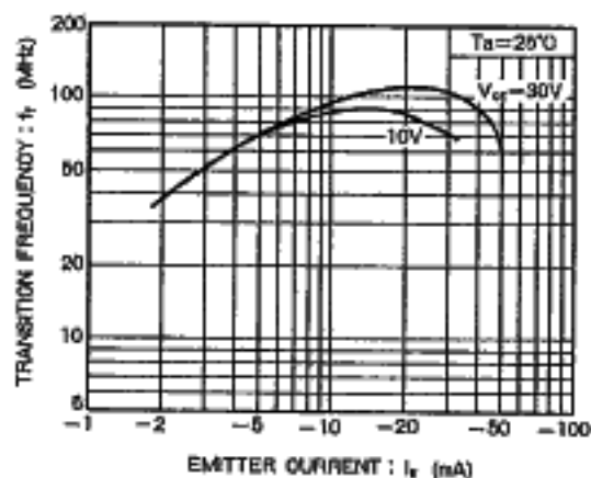
Fig. 10 利得帯域幅積—エミッタ電流特性
