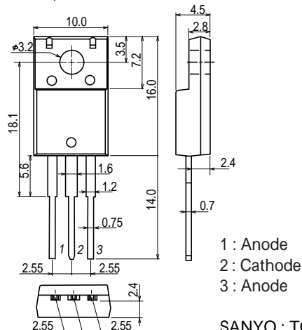
外形図 1320 (unit : mm)
