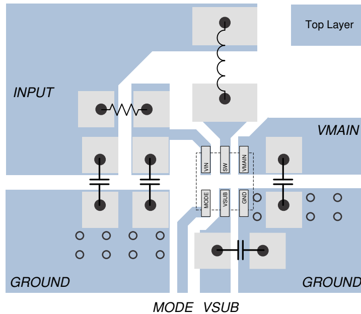
图 11-1. Layout
