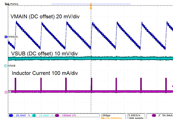
图 9-4. Switching Waveforms
