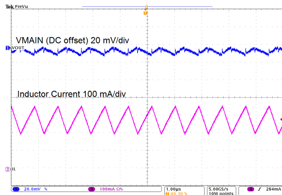
图 9-3. Switching Waveforms
