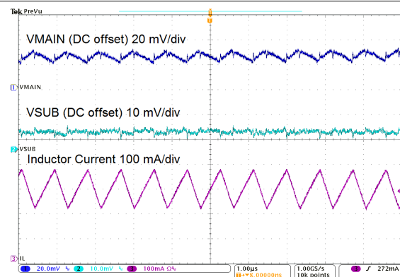
图 9-6. Switching Waveforms
