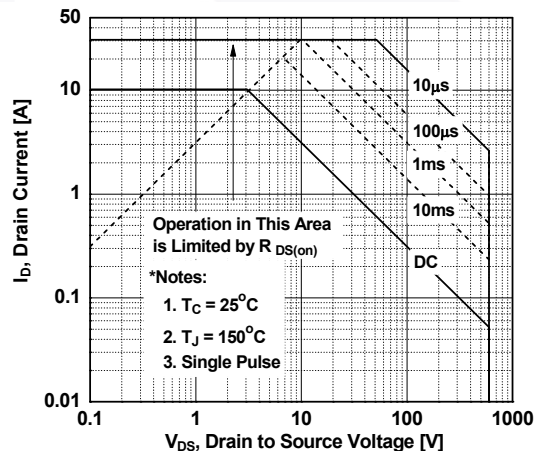
图 10. 最大安全操作区 (FCPF380N60E)
