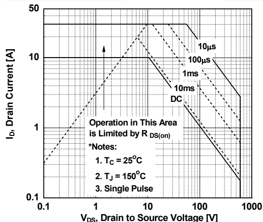
图 9. 最大安全工作区(FCP380N60E)
