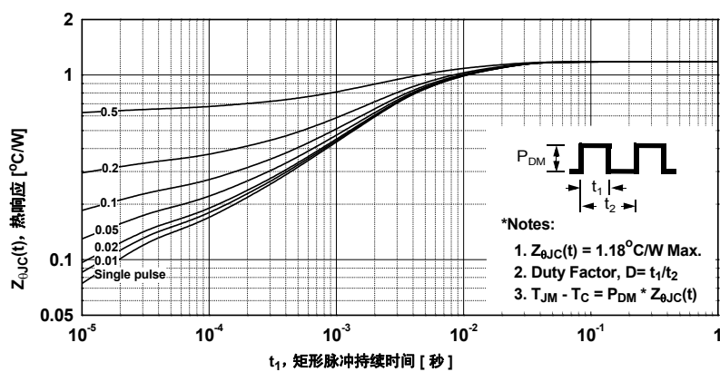
图 14. 瞬态热响应曲线 (FCPF380N60E)
