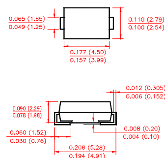
DO-214AC(SMA)
