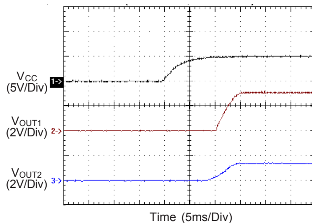
POR (Start Up)
