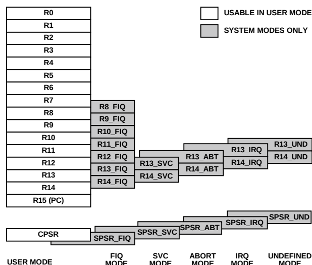
图34. 寄存器结构图
