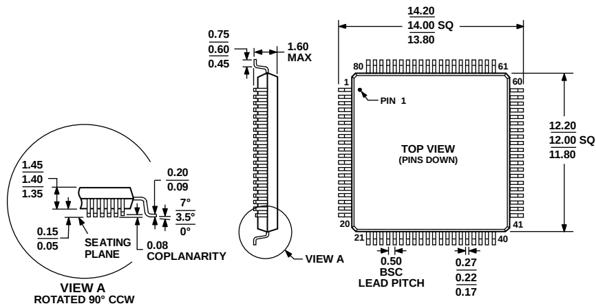
图87. 80引脚薄型四方扁平封装[LQFP]
