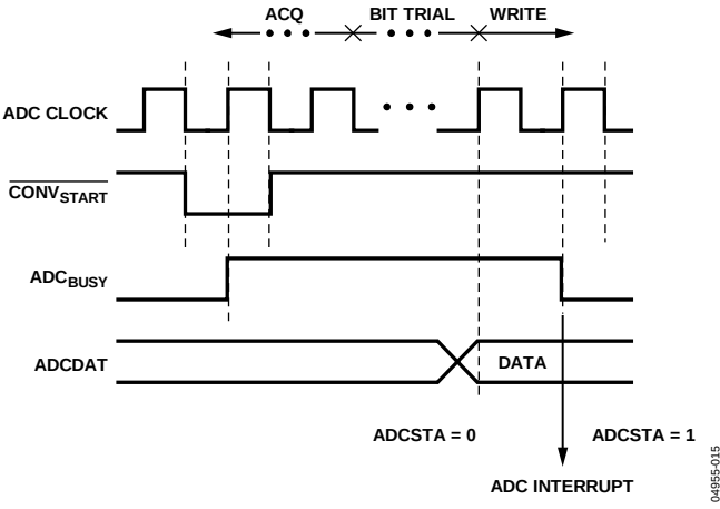
图42. ADC时序
