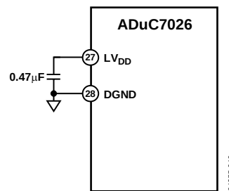
图78. 稳压器连接
