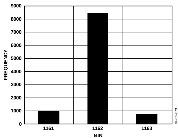
图24. f_s = 774 \text{ kSPS} 、 V_{IN} = 0.7 \text{ V} 时代码直方图
