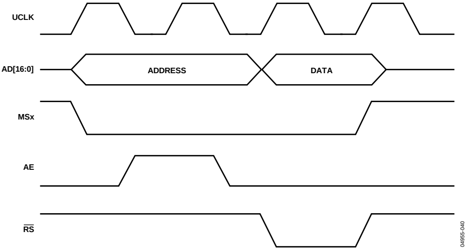
图71 外部存储器读周期
