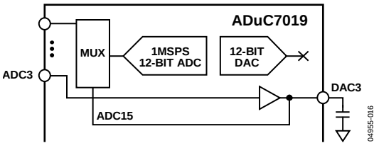
图43. ADC3缓冲输入
