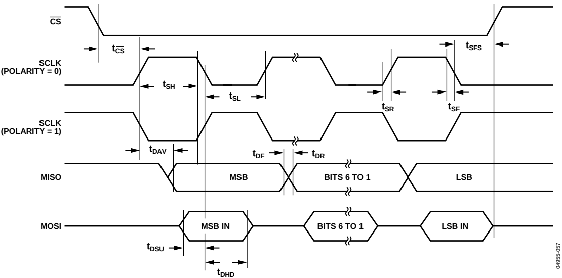
图8. SPI从机定时(相位模式 = 1)
