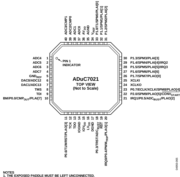
图 11. ADuC7021 40引脚LFCSP_VQ封装引脚配置
