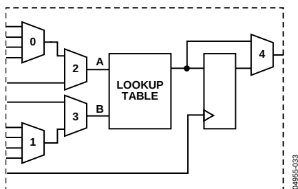
图64. PLA单元
