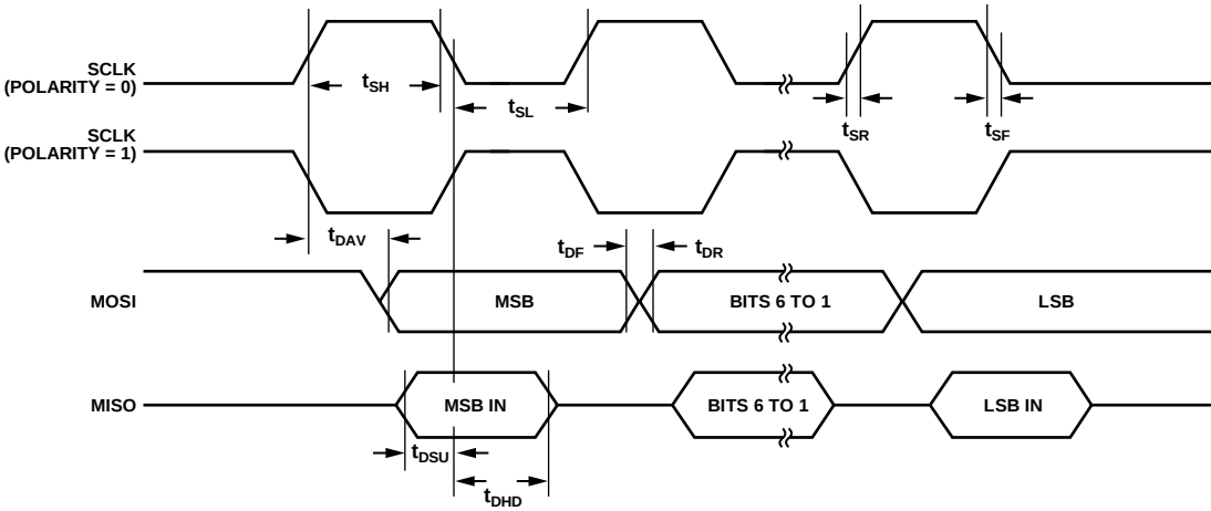
图6. SPI主机定时(相位模式 = 1)
