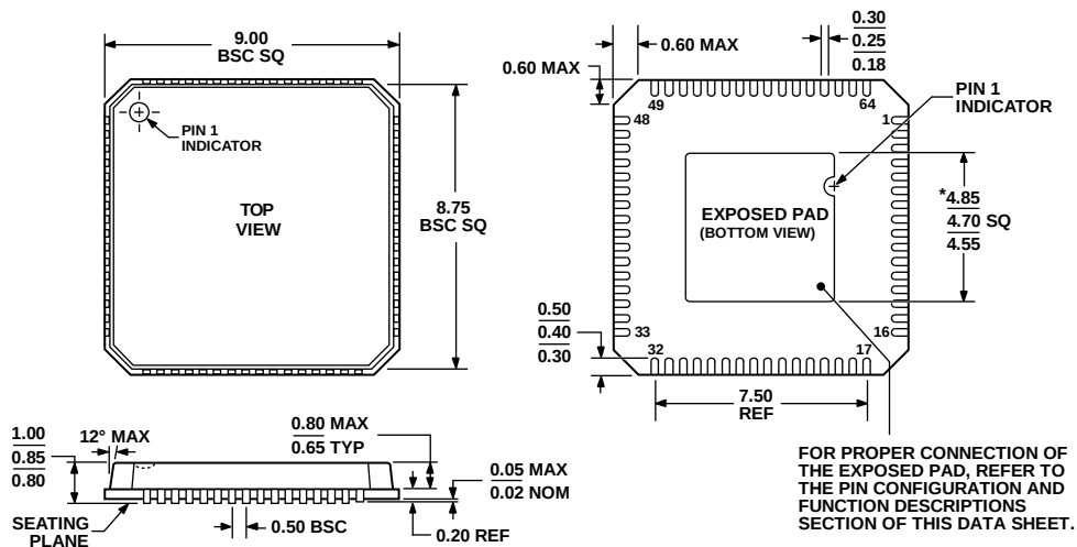
图85. 64引脚|脚架构芯片级封装[LFCSP_VQ]
