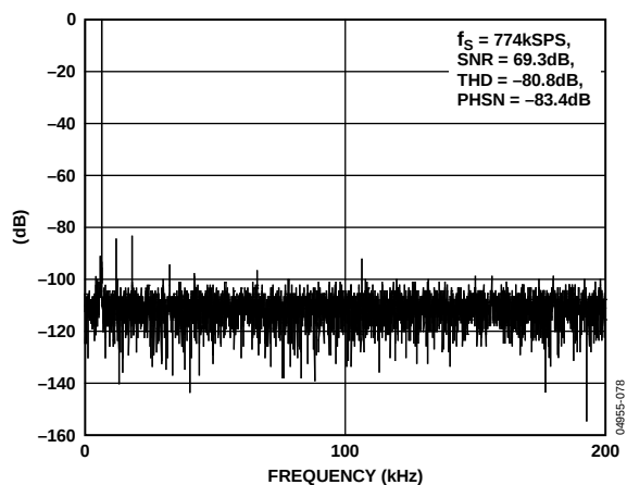
图25. f_s = 774 \text{ kSPS} 时动态性能
