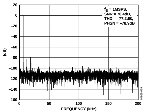
图26. f_s = 1 \text{ MSPS} 时动态性能
