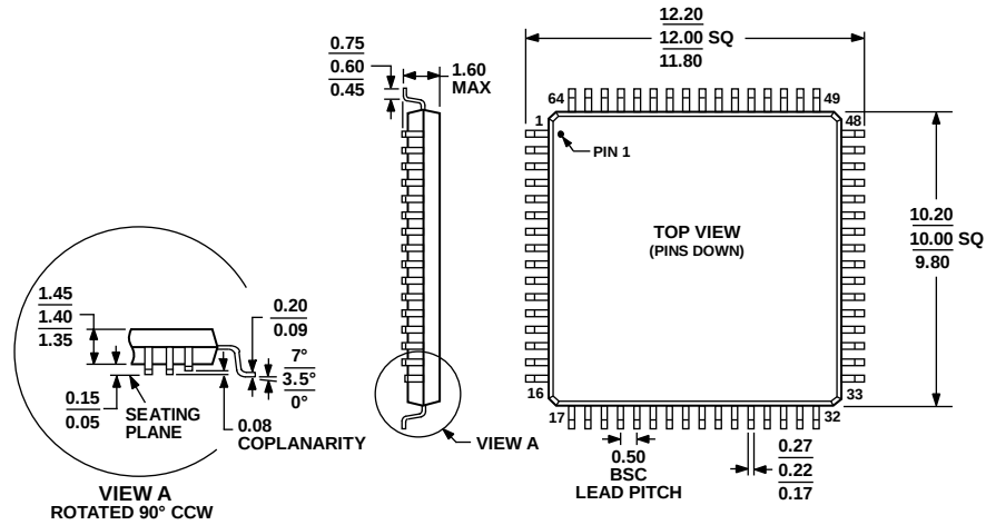
图86. 64引脚薄型四方扁平封装[LQFP]
