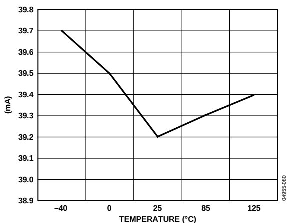
图29. CD = 0 时功耗与温度的关系
