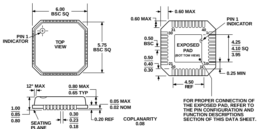
图84. 40引脚|脚架构芯片级封装[LFCSP_VQ]
