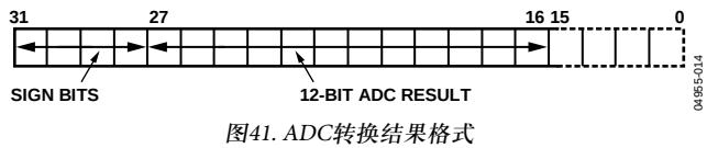
图41. ADC转换结果格式
