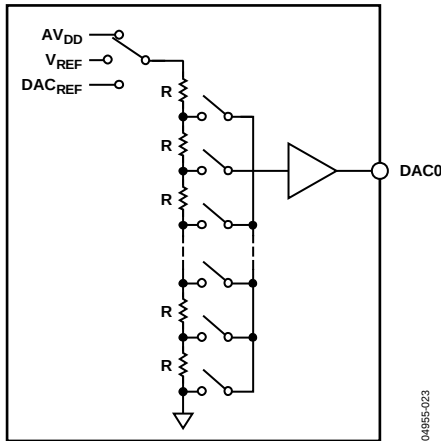
图53. DAC结构
