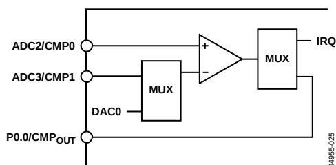
图55. 比较器
