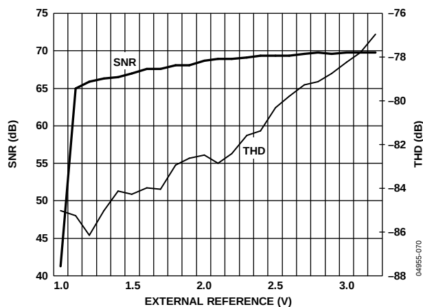
图27.典型动态性能与 V_{REF} 关系
