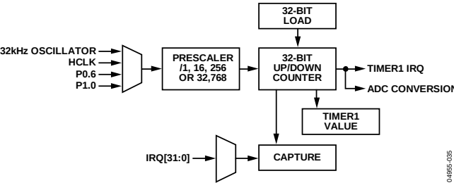
图66. 定时器1框图
