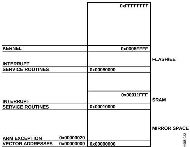
图52. 异常重映射
