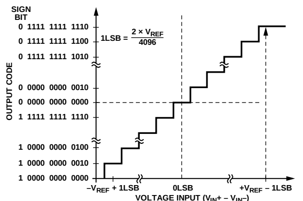
图40. 差分模式下ADC传递函数
