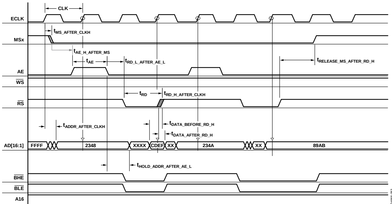
图4. 外部存储器读周期(参见表78)
